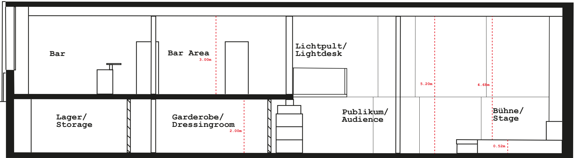
Schnitt Bar/ Sideview Bar
